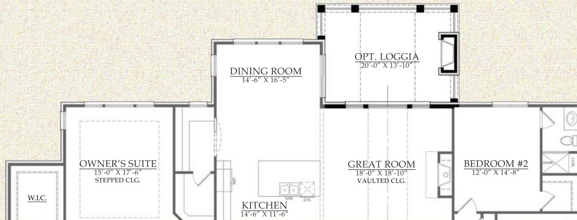
OPTIONAL LOGGIA PLAN
